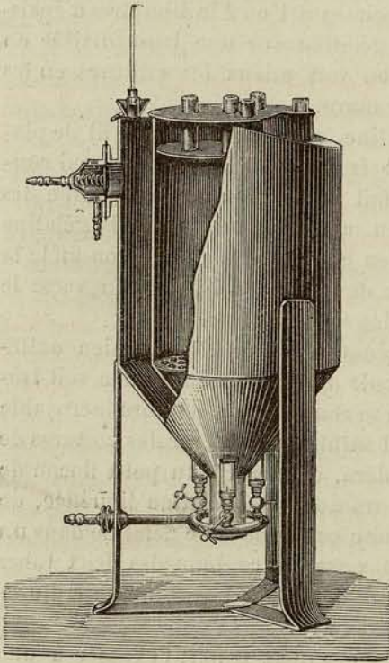
Fig. 18. — Étuve de d'Arsonval.
