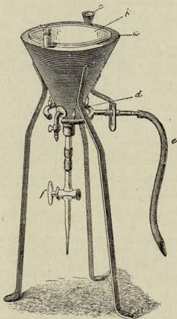
Fig. 12. — Filtre pour la gélatine peptone fabriqué par Wisnegg.
