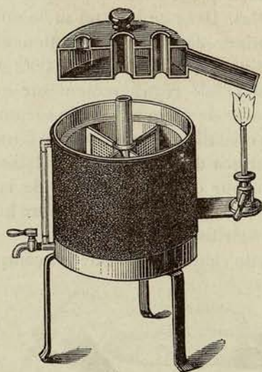
Fig. 16. — Appareil pour chauffer les tubes contenant du sérum (d'après Koch, figure de Muencke).
