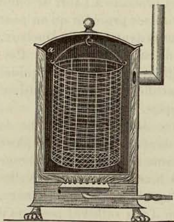
Fig. 5. — Coupe du chauffeoir employé pour flamber et stériliser les instruments et la verrerie.
